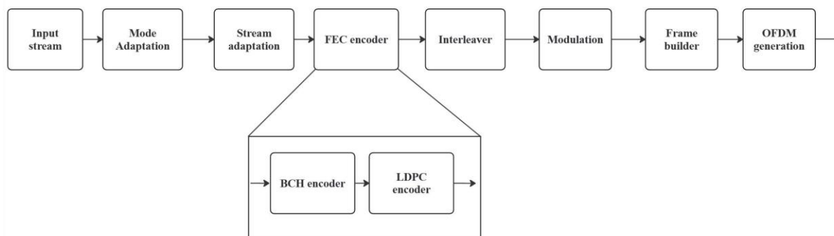
Рис. 2] Структурная схема системы DVB-T2.
